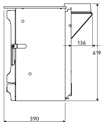
CÔTÉ
