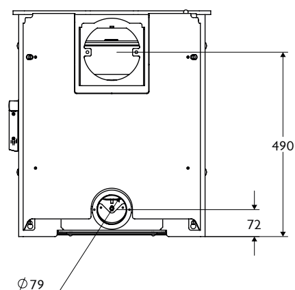
DERRIÈRE
