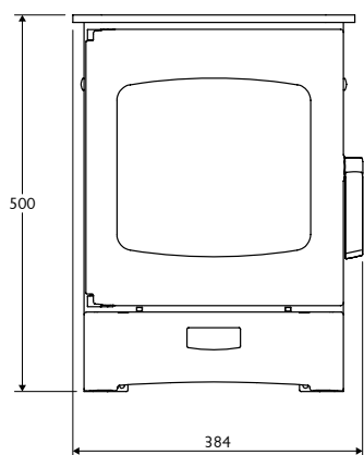
DEVANT
