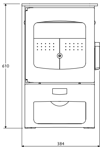
MODÈLE BÛCHER
