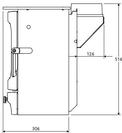
CÔTÉ
