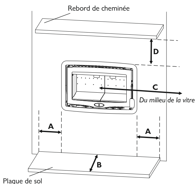
Fig. 9 Distances minimales avec les matériaux combustibles
