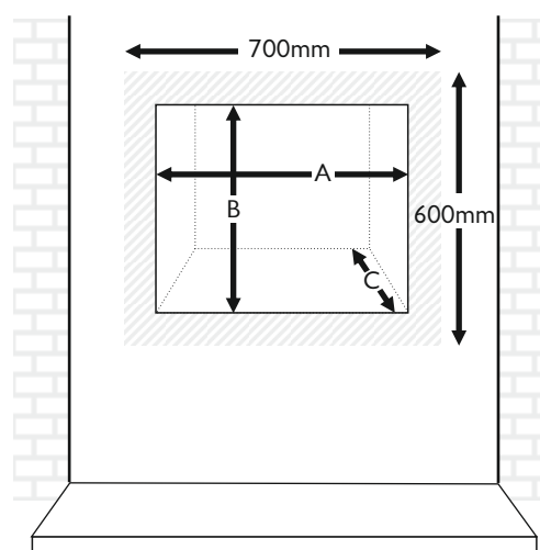
Fig. 11 Dimensions minimales du pourtour et ouverture
