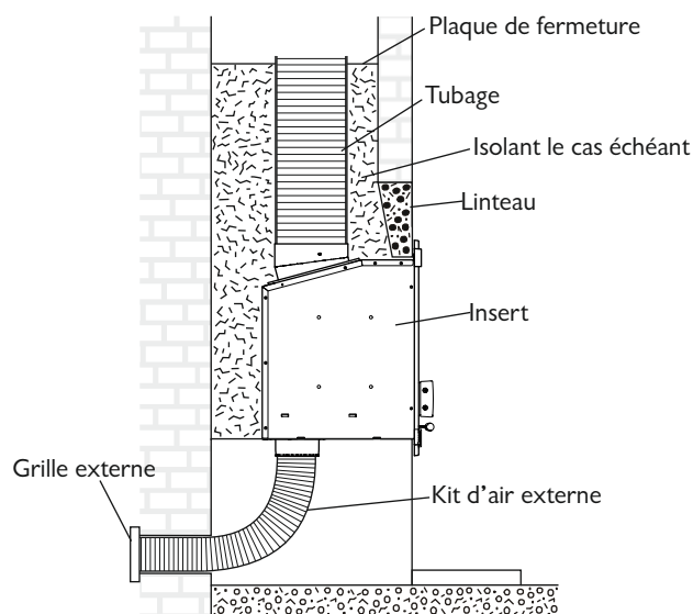
Fig. 12 Installation dans une cheminée standard non combustible. (non applicable pour la France)
