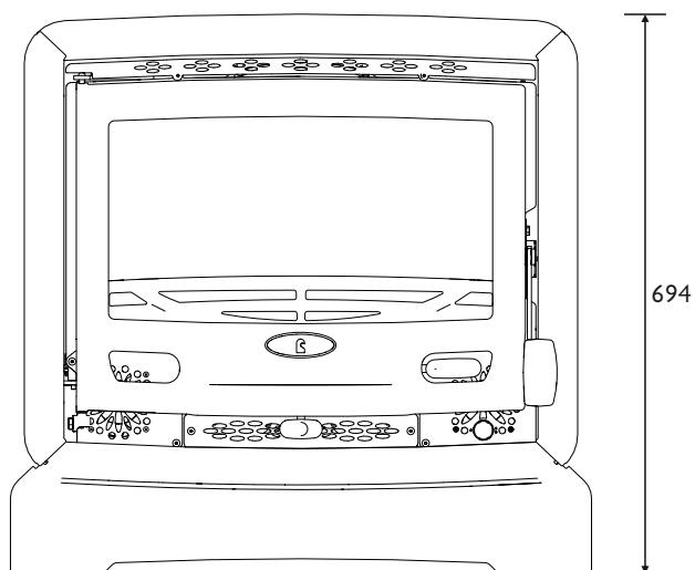
VUE DE FACE AVEC PLINTHE DÉCORATIVE
