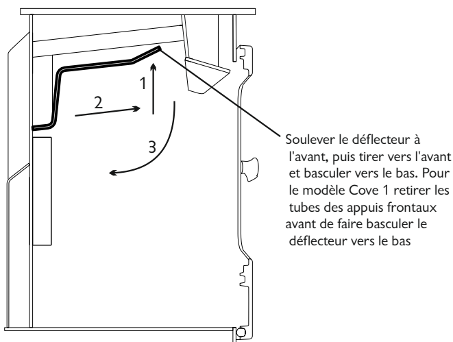
Fig. 4. Déflecteur
