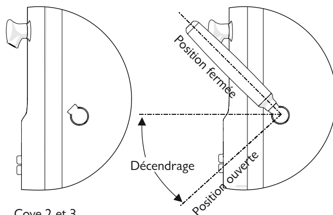
Fig. 2. Grille de décendrage
