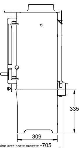
VUE LATÉRALE
