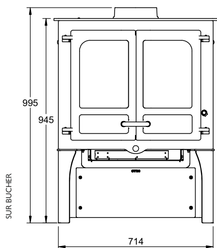
VUE AVANT
