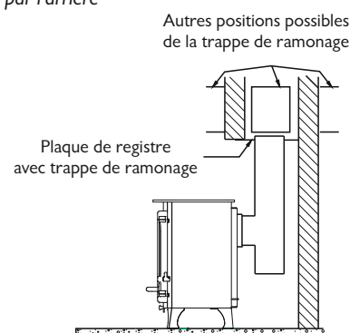
Fig. 10. Plaque de registre horizontale avec branchement de conduit de fumée par l'arrière
