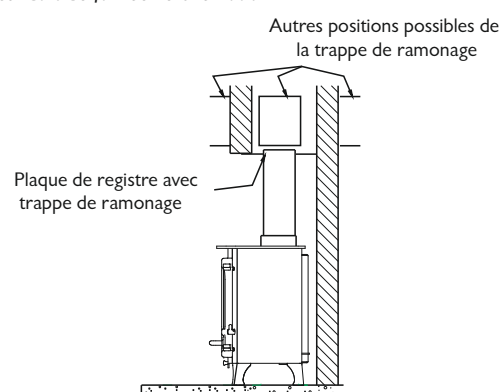
Fig. 12. Plaque de registre horizontale avec raccordement de fumées vertical arrière en option
