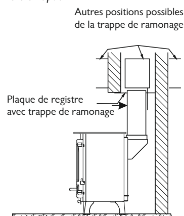
Fig. 12. Plaque de registre horizontale avec raccordement de fumées vertical arrière en option
