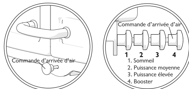
Fig. 3 Contrôle de l'air
