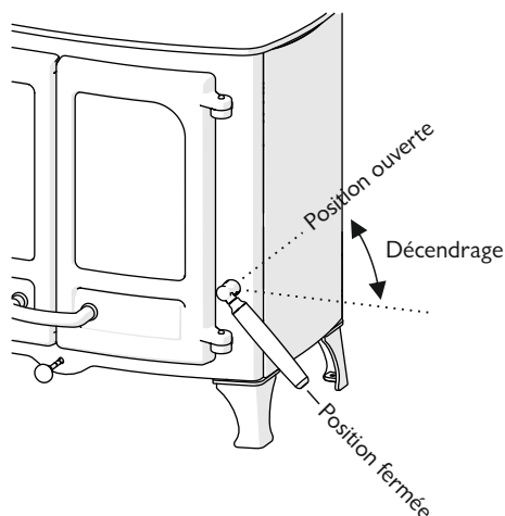
Fig. 2. Grille de décendrage
