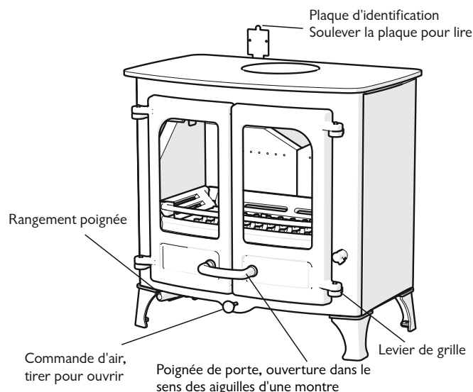
Fig. 1. Commandes du poêle
