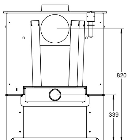
VUE ARRIÈRE
