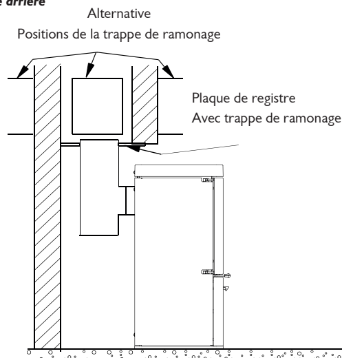
Fig.8 Fig. 6 Plaque de registre horizontale avec raccordement au conduit de fumée arrière
