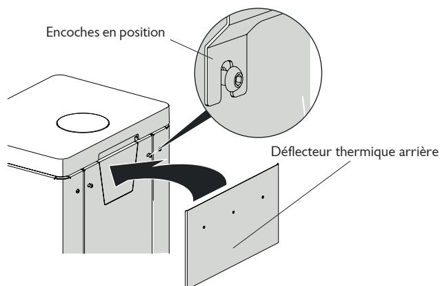
Fig. 13. Montage du déflecteur thermique arrière
