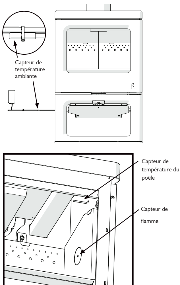
Fig. 4 Capteurs
