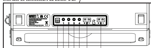
Interface de connecteurs du boîtier d'air
