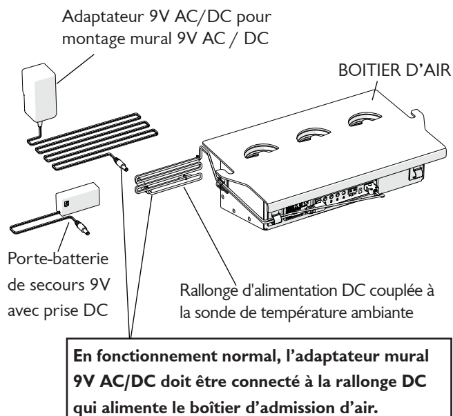
Fig. 19 Connexions électriques
