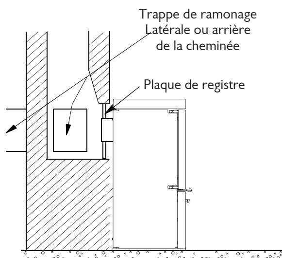
Fig.7 Plaque d'enregistrement verticale avec cheminée en brique
