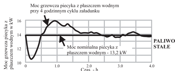
Rys.4. Wykres wydajności
