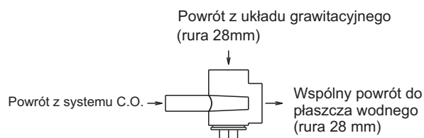
Rys. 7. Trójnik
